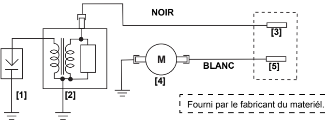
DÉMARREUR ÉLECTRIQUE (à frein-embayage)
