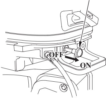
CHOKE KNOB
