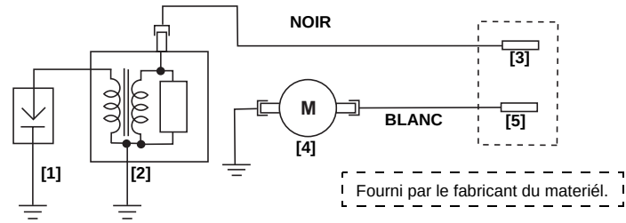
DÉMARREUR ÉLECTRIQUE (à frein-embrayage)
