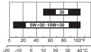
OMGEVINGSTEMPERATUUR
