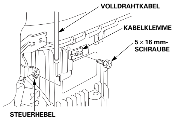
STEUERHEBEL
