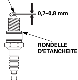
ELECTRODE LATÉRALE
