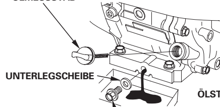
ÖLEINFÜLLVERSCHLUSS/ ÖLMESSTAB
