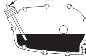
ÖLEINFÜLLVERSCHLUSS/ ÖLMESSTAB
