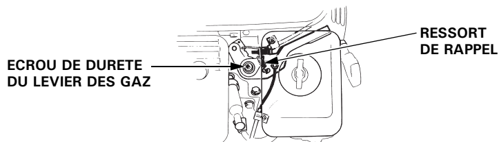
Fixation de câble à âme flexible
