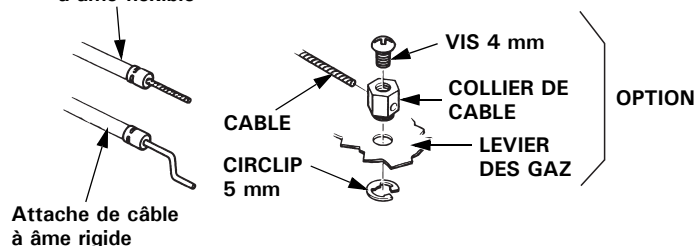
Fixation de câble à âme flexible
