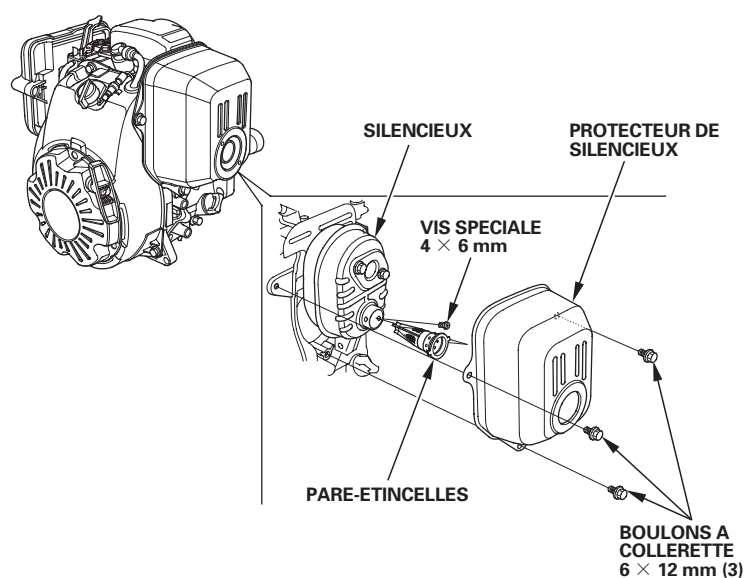
GRILLE DE PARE-ÉTINCELLES
