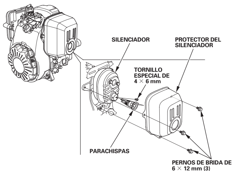
PANTALLA PARACHISPAS
